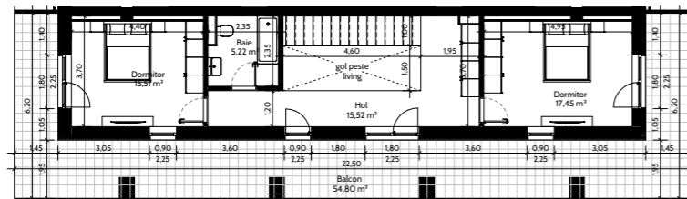
PLAN ETAJ
